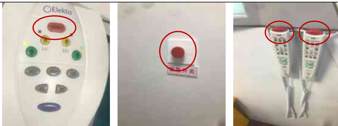
图3-4 急停按钮
