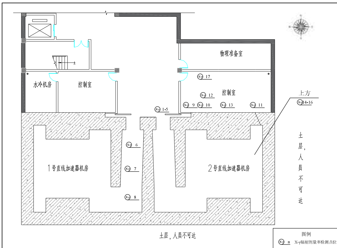
图7-1 2号直线加速器机房周围X-γ辐射剂量率监测布点图
