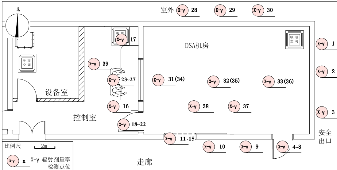
图7-1 本项目DSA机房周围X-γ辐射剂量率监测布点图
