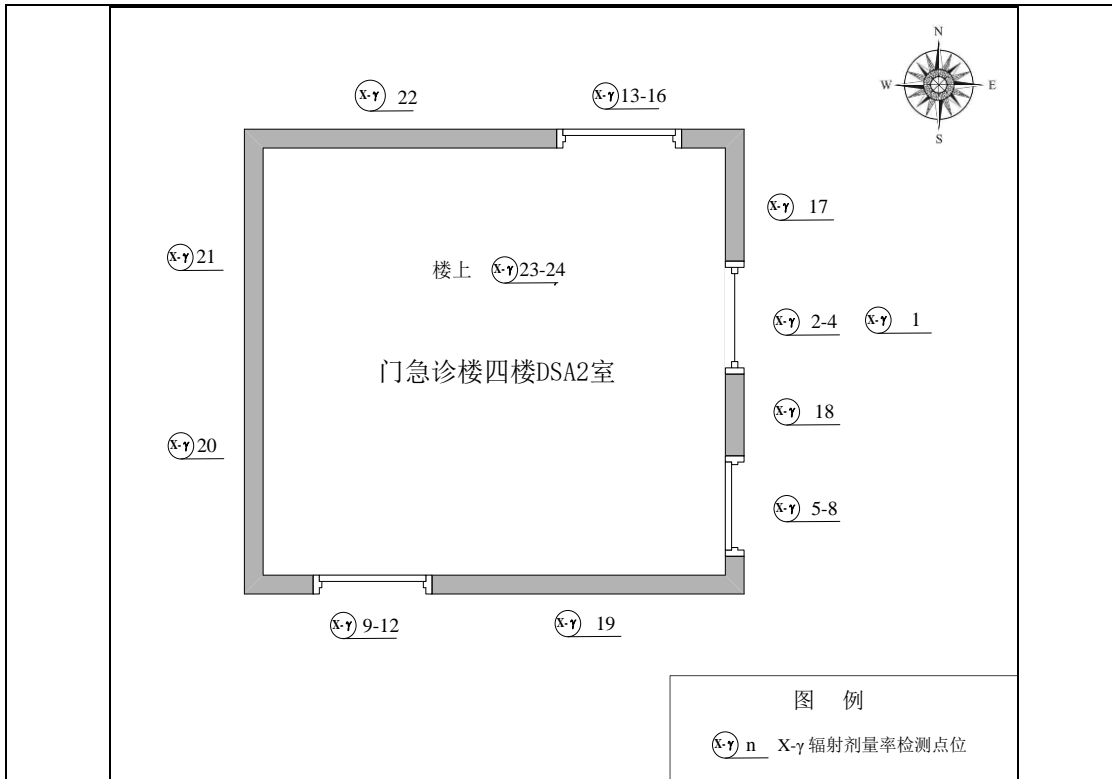
图7-2 门急诊楼四楼DSA2室周围监测布点图
