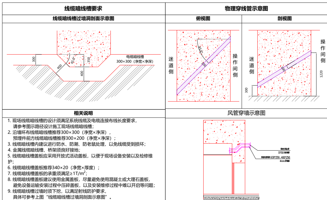
图 10-3 直线加速器机房电缆沟、物理管线和风管穿墙示意图
