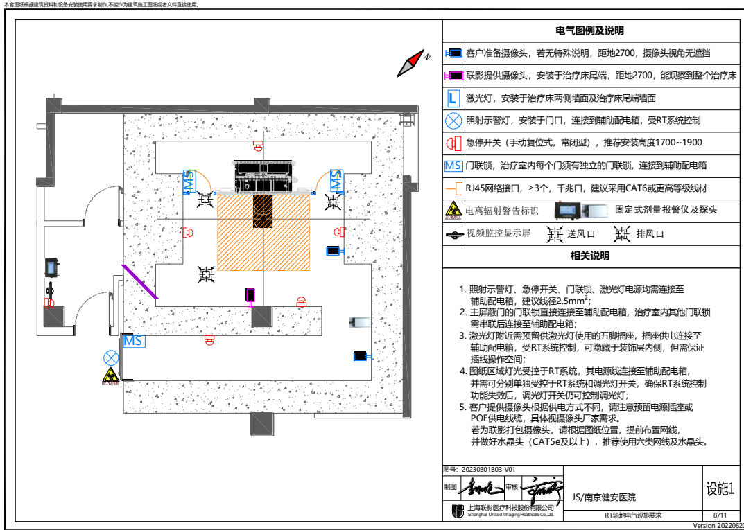
图 10-2 医用直线加速器机房主要安全设施位置示意图
