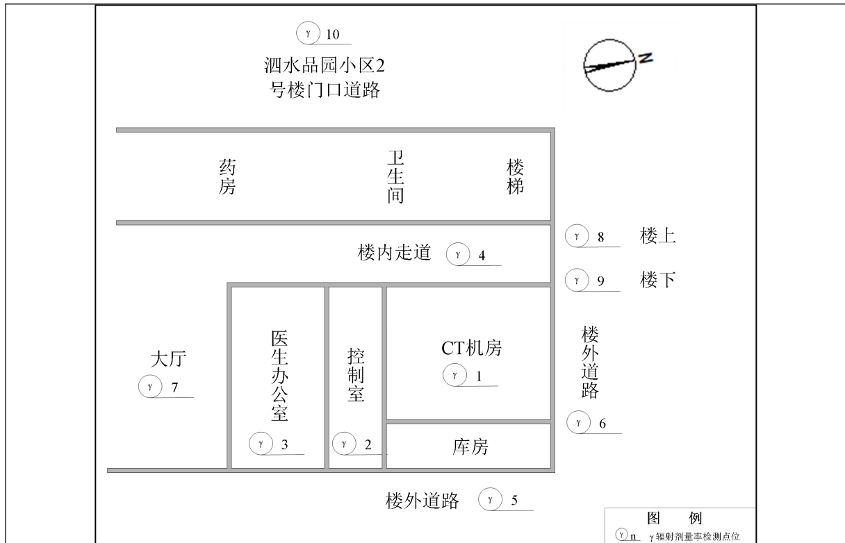
图 8-8 泗阳县中医院有限公司新增 1 台、搬迁 1 台 DSA 项目拟建址周围 \gamma 辐射监测点位示意图
