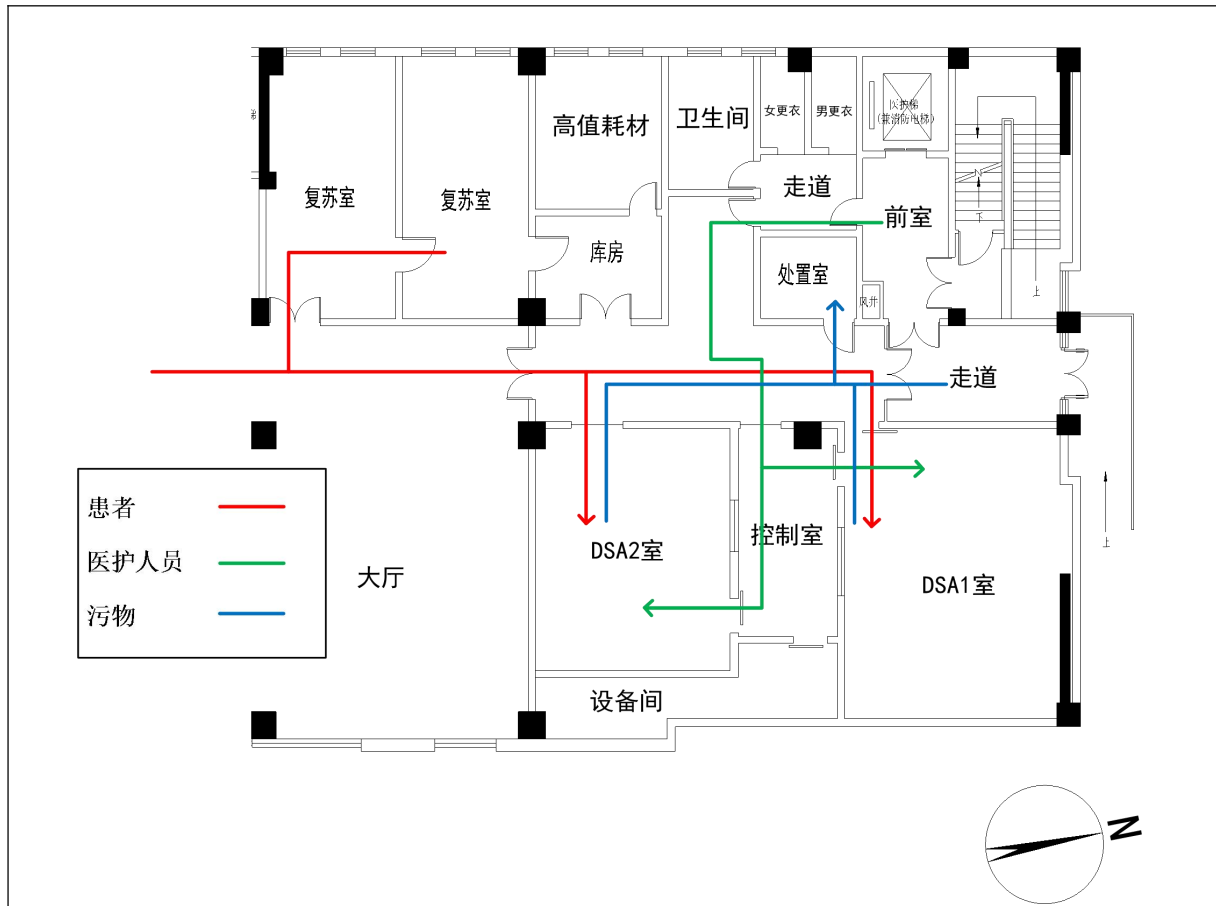
图 10-2 本项目患者、医护人员及污物路线示意图
