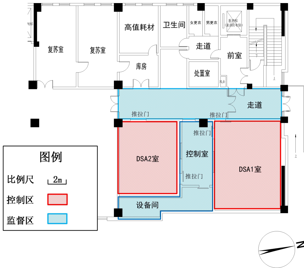
图 10-1 本项目 DSA 机房周围布置及分区示意图
