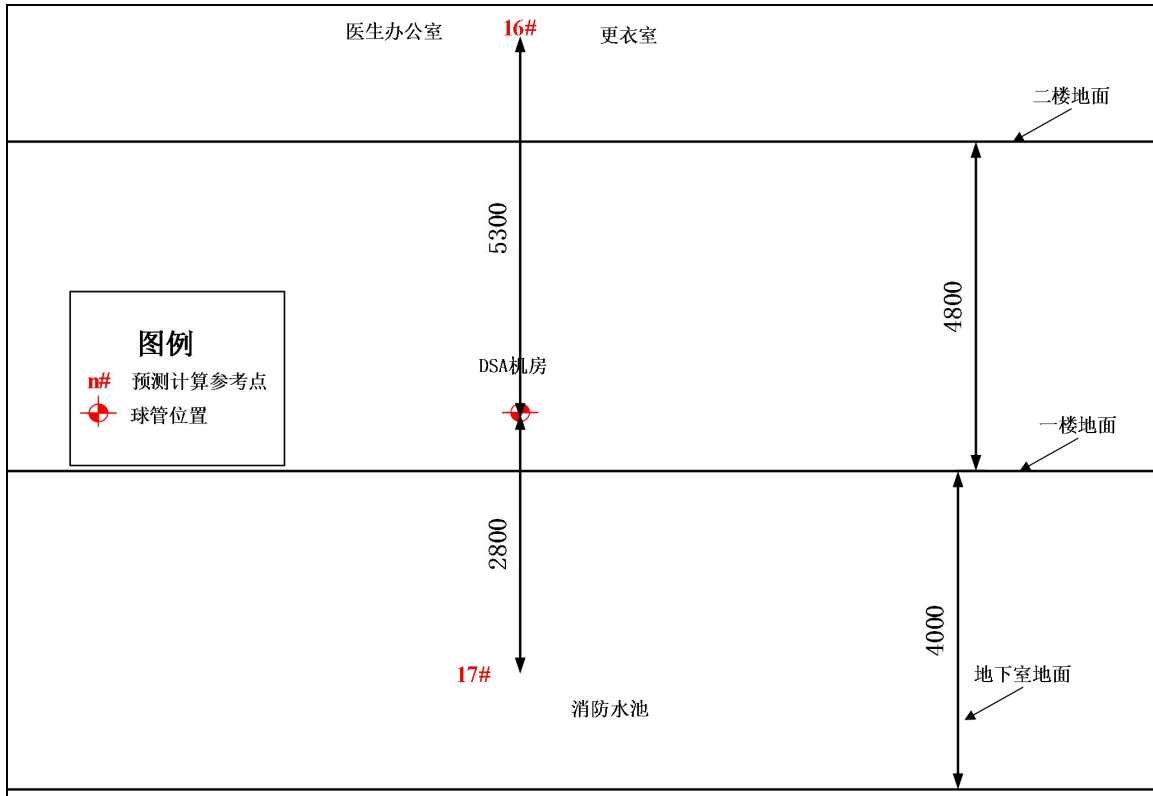
图 11-2 DSA 机房预测点布设剖面示意图
