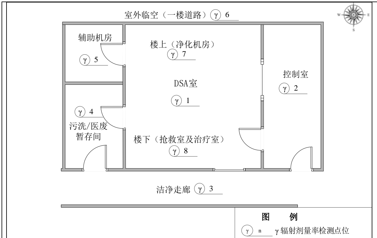
图 8-8 南京市江宁医院新增 1 台 DSA 项目拟建址周围环境 \gamma 辐射监测点位示意图
