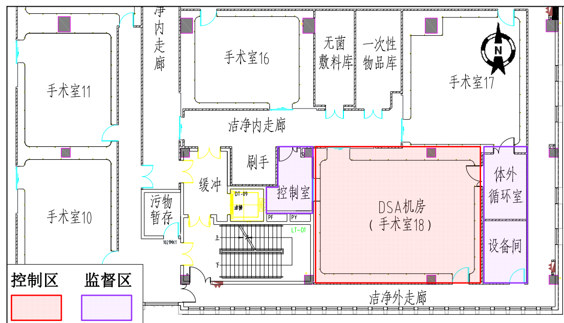
图3-1 如东县人民医院外科大楼四层DSA机房平面布置及分区示意图
