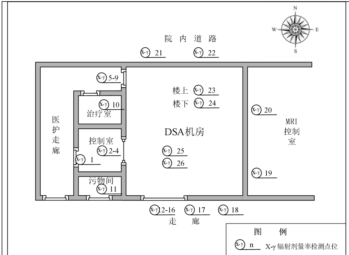
图7-1 本项目影像科DSA机房周围X-γ辐射剂量率监测布点图
