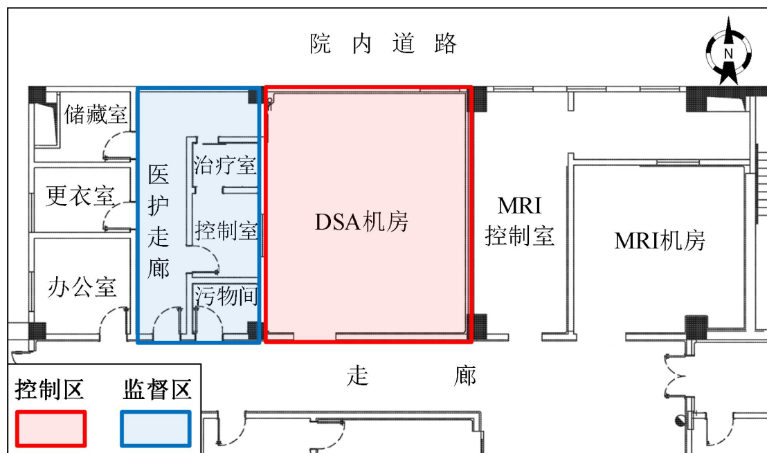
图3-1 如东县人民医院门急诊大楼一层DSA机房平面布置及分区示意图
