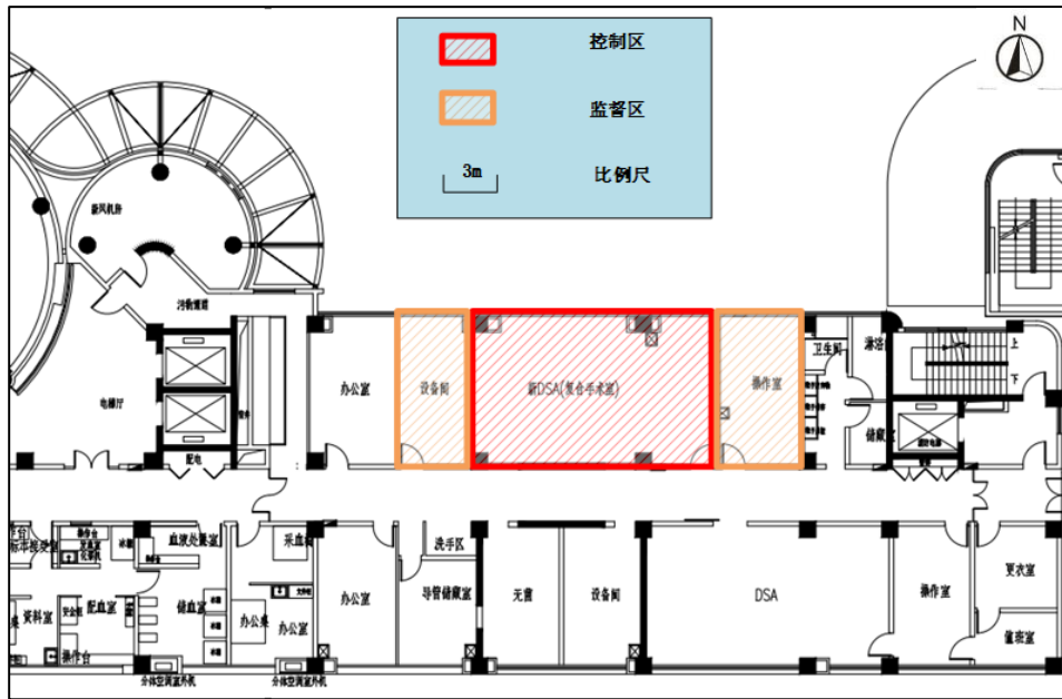
图3-1 北院区住院部二楼介入手术室二平面布置及分区示意图
