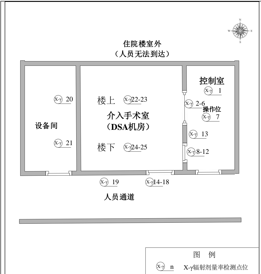
图7-1 住院部二楼介入手术室二周围监测布点图
