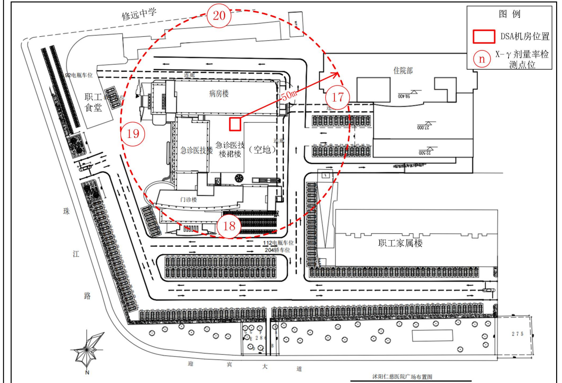
图 7-1 DSA 机房周围 X-γ辐射剂量率现场检测点位示意图
