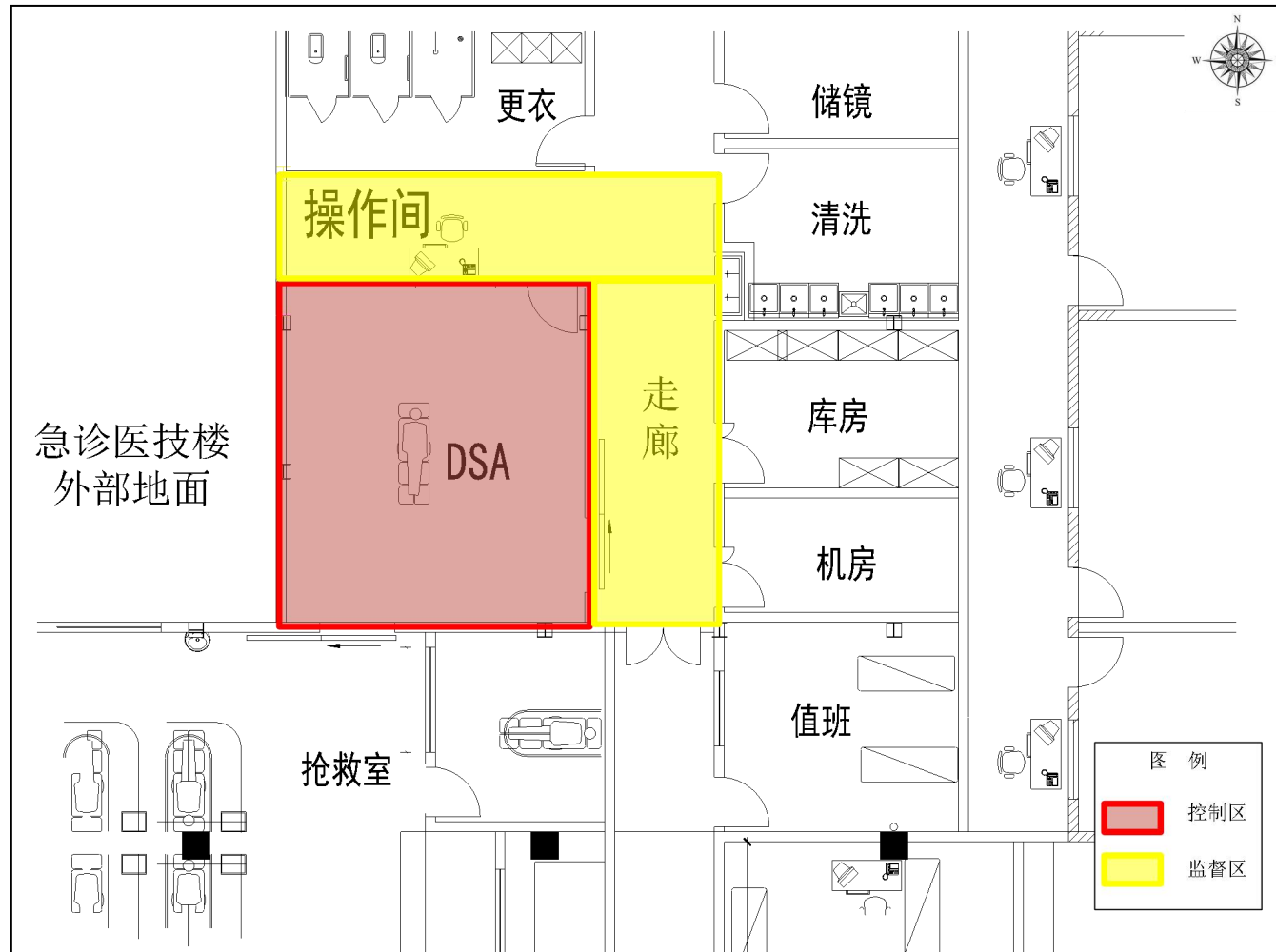
图3-2 本项目工作场所平面布置及两区划分示意图
