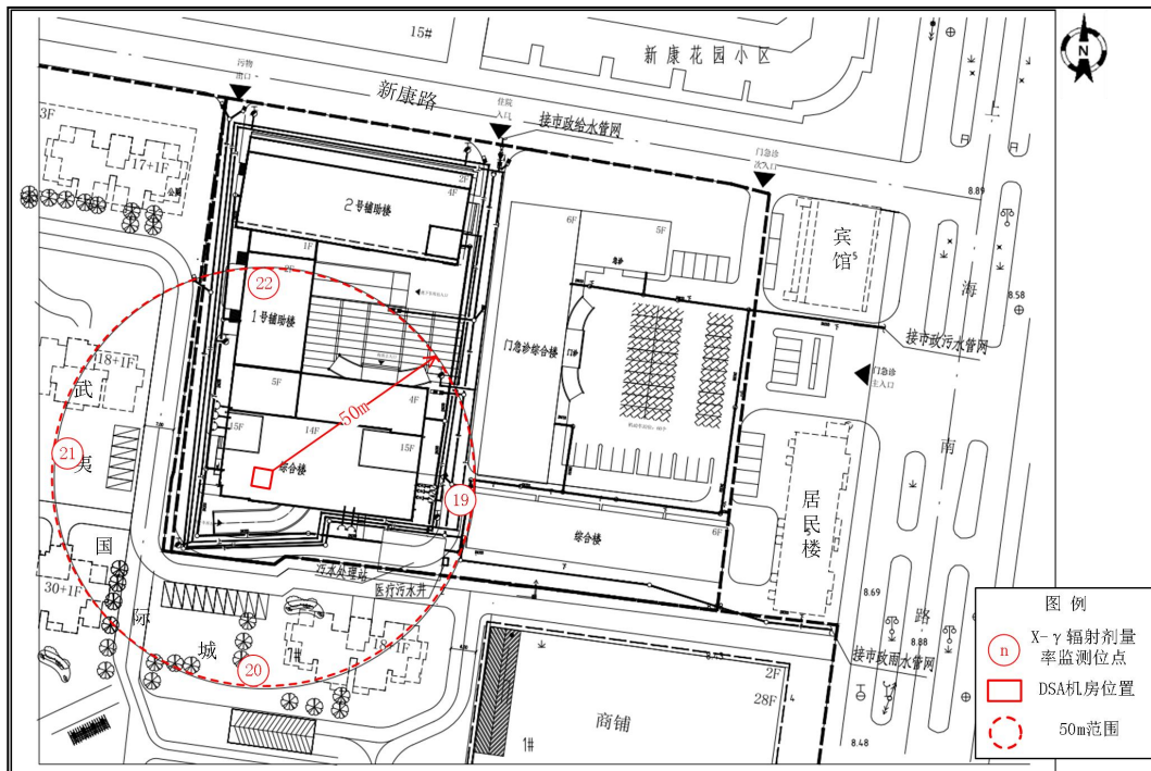
图 7-2 DSA 机房周围 X-γ 辐射剂量率现场检测点位示意图
