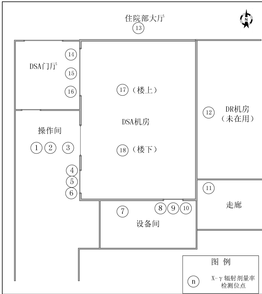
图 7-1 DSA 机房周围 X-γ 辐射剂量率现场检测点位示意图
